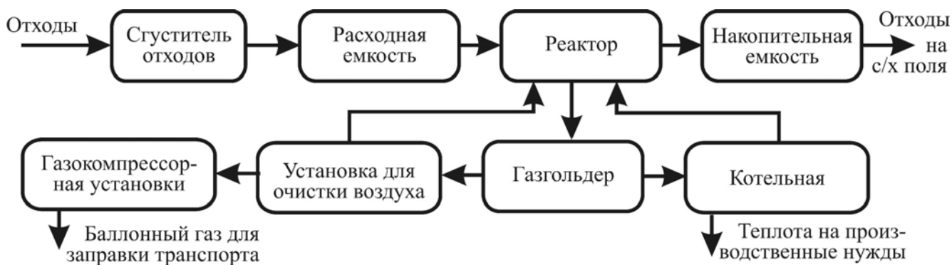
Рисунок 1.1. Схема энергокомплекса с биогазовой установкой и газокomppressorной станцией для крупных сельскохозяйственных предприятий [1]
