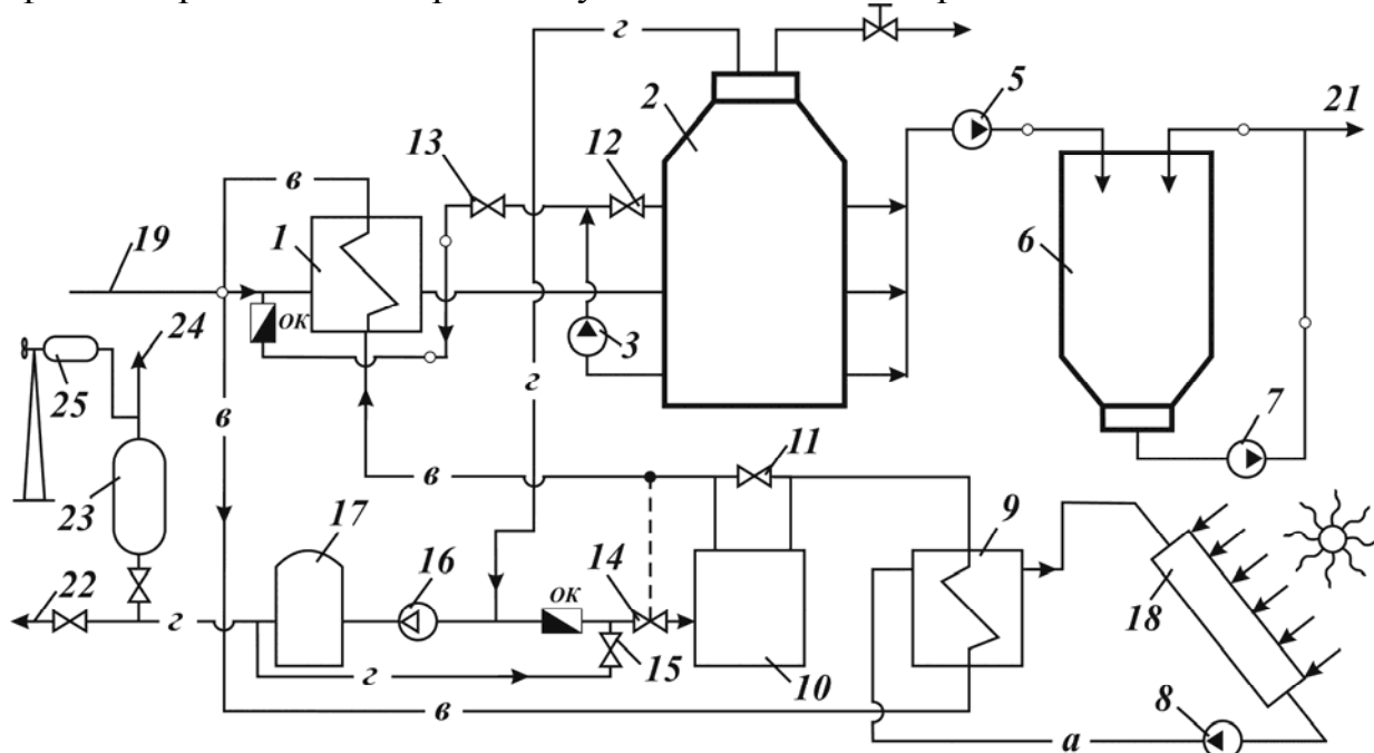
Рисунок 1.2. Комбинированная солнечно-биогазовая установка: 1, 9 – теплообменники; 2 – метантенк; 3, 5, 7, 8 – насосы; 4 – предохранительный клапан; 6 – отстойник; 10 – котел; 11, 13, 12, 15 – вентиля; 14 – регулирующий клапан; 16 – компрессор;
