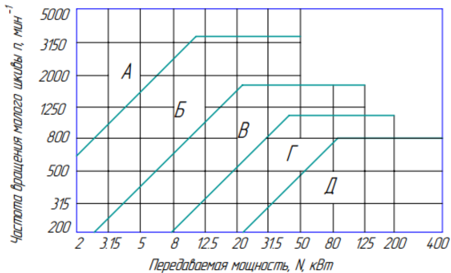
Рисунок 2 - Номограмма определения требуемого сечения ремня
