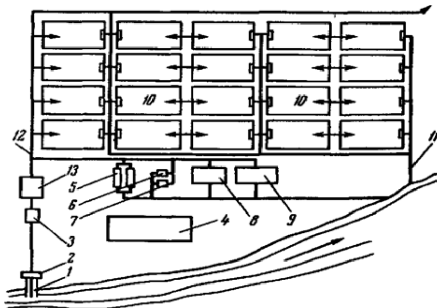
Рис. 1 Схема лососевого рыбоводного завода:
