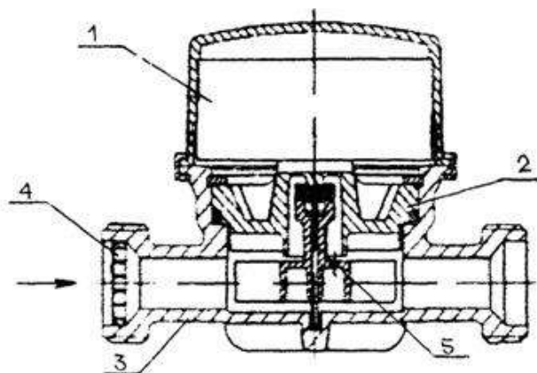
Рисунок 3 Конструкция счетчика вихревого типа: 1 - поворачивающийся счетный механизм; 2 – пластина, отделяющая счетный механизм от водяной камеры; 3 - корпус; 4 - фильтр; 5 - тело обтекания.
