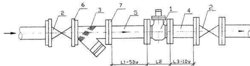
Рисунок 2 Схема монтажа: 1 - счетчик воды; 2 - задвижка; 3 - фильтр магнитный; 4 - патрубков; 5 - патрубков; 6 - прокладка; 7 - фланец по ГОСТ 12815.
