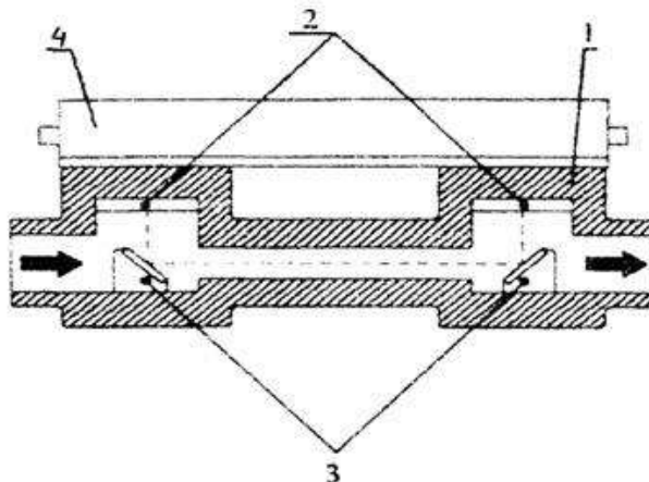
Рисунок 5 Конструкция счетчика ультразвукового типа: 1 - корпус; 2 - преобразователи ультразвука; 3 - отражатели; 4 - электронный блок.
