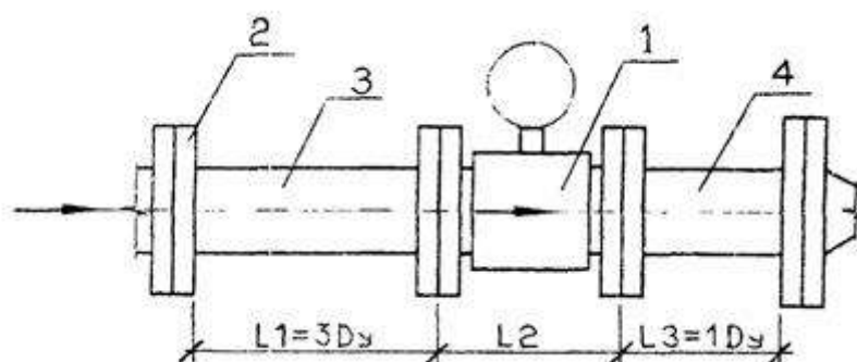
Рисунок 8 Схема монтажа: 1 - электромагнитный счетчик; 2 - фланец; 3, 4 – патрубок
