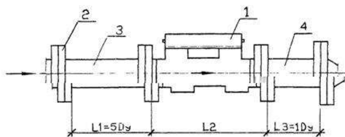
Рисунок 6 Схема монтажа: 1 - ультразвуковой счетчик; 2 - фланец; 3, 4 – патрубок.
