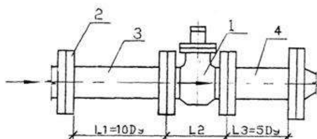
Рисунок 4 Схема монтажа: 1 - счетчик воды; 2 - фланец по ГОСТ 12815; 3 - патрубков; 4 – патрубков.
