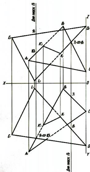
Рис. 4. Построение точки K' —точки встречи прямой AB с плоскостью S(DEL) и нахождение линии пересечения плоскостей R(ABC) и S(DEL)
