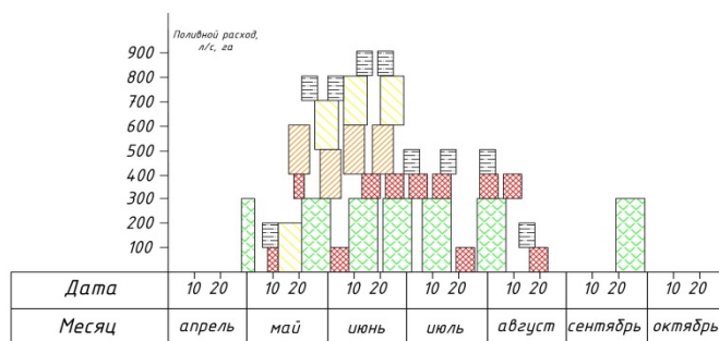
Неукомплектованный график поливных расходов
