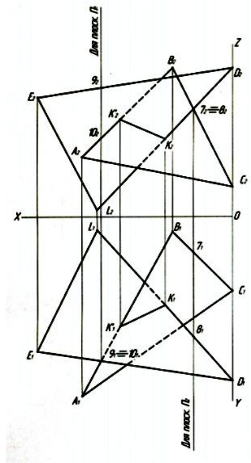
Рис. 5. Определение видимости сторон треугольников (ABC) и (DEL)
