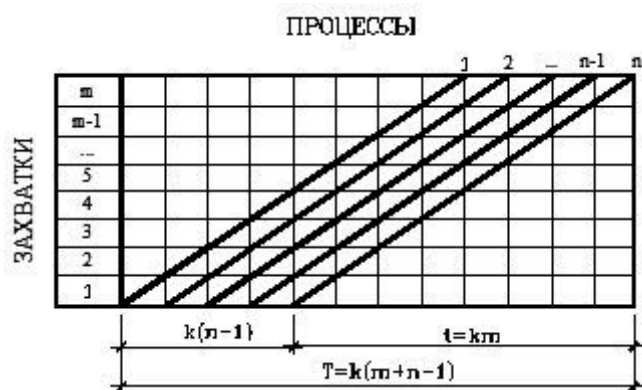
Рис. 1 - Циклограмма строительного потока
