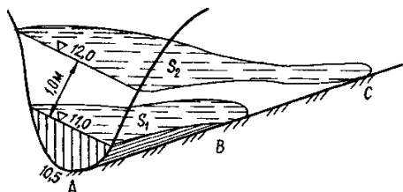
Рис. 2. Схема расчетных объемов пруда
