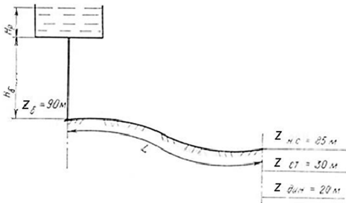
Рисунок 1 – Расчетная схема подачи воды
