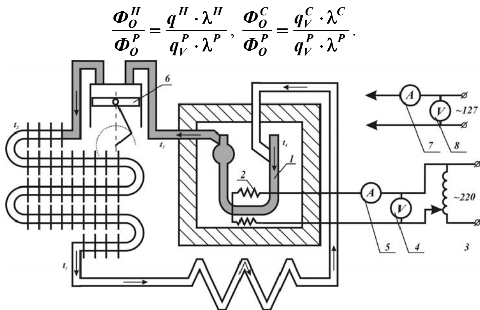
Рис. 4. Установка для изучения цикла холодильных машин
