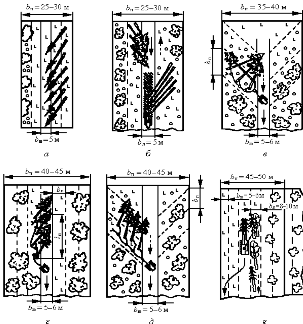
Рис. 1. Технологические схемы разработки пасек при заготовке на лесосеке деревьев и хлыстов бензиномоторными пилами:
