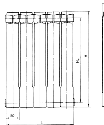
Рисунок 5 - Габаритные размеры радиатора «Сантехпром БМ»
