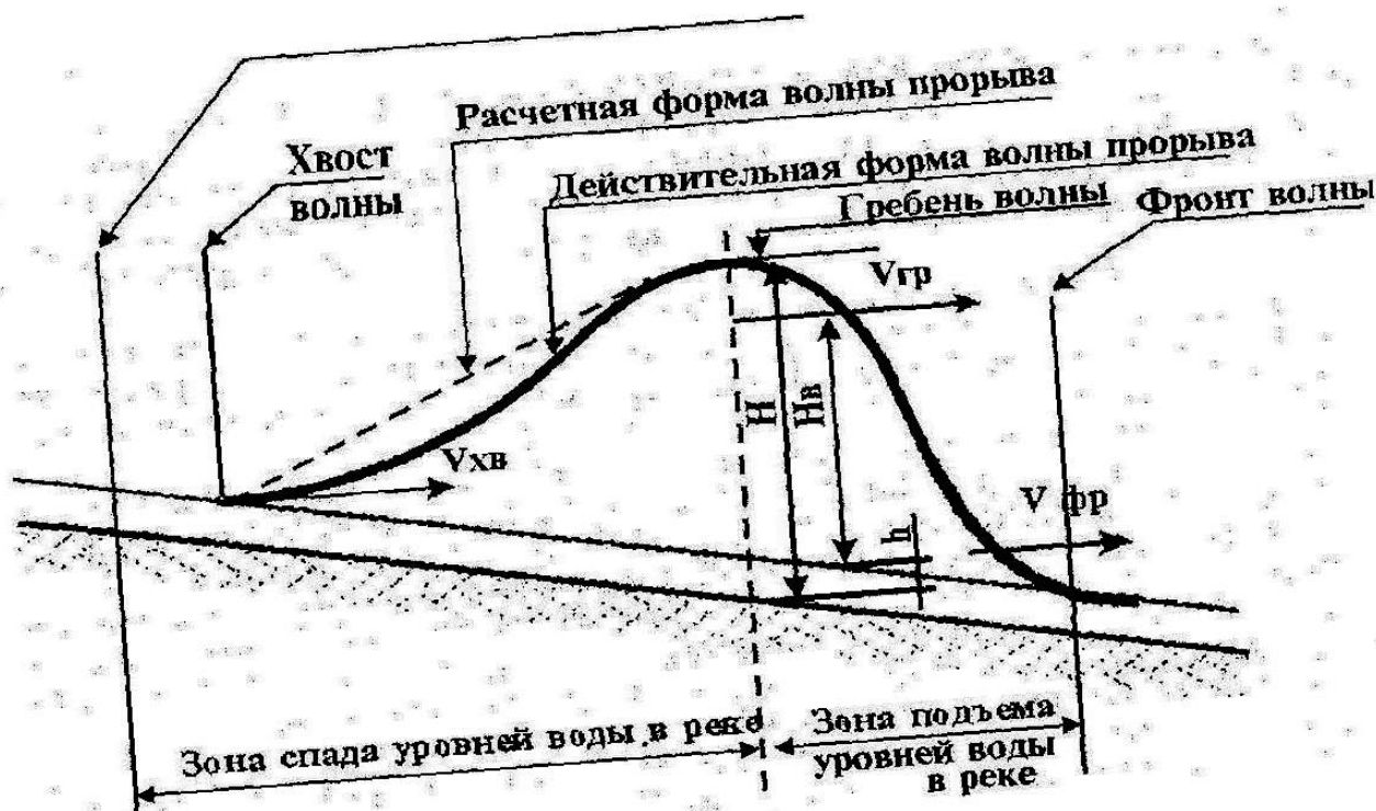
Рисунок 1. Схематический продольный разрез волны прорыва
