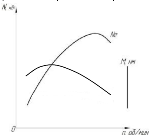
Рис. 1. График внешней скоростной характеристики двигателя
