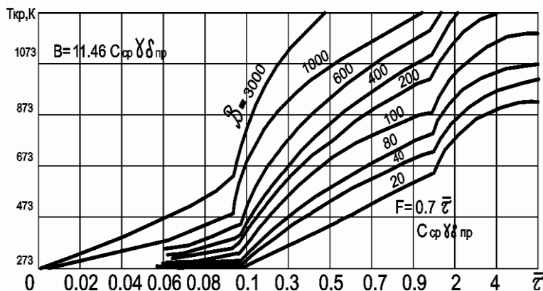
Рис. 1 Номограмма для расчета огнестойкости незащищенных металлических конструкций
