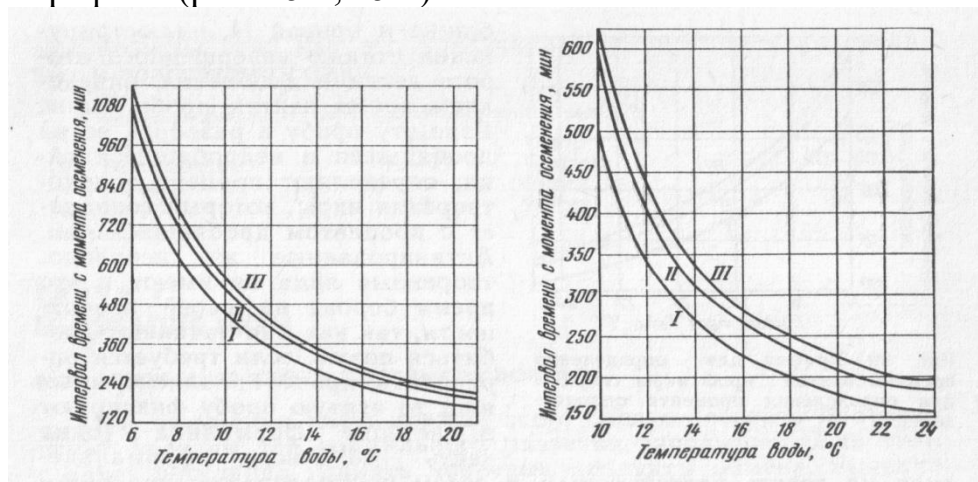
Рисунки 15.1, 15.2. Графики для определения времени взятия проб икры белуги и осетра для определения процента оплодотворения
