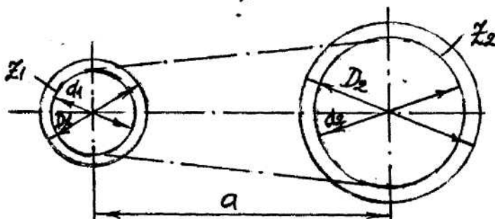
Рисунок 3.3. Расчётная схема передачи
