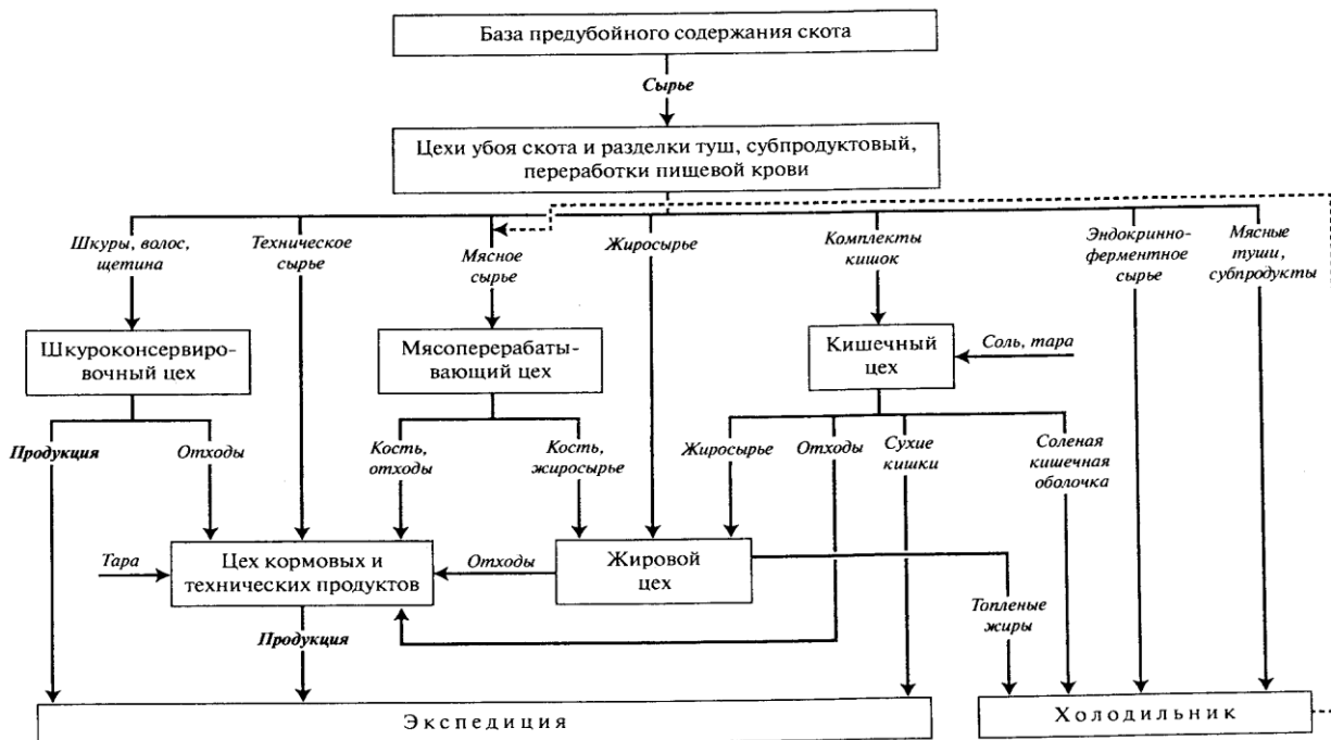
Рисунок 1 – Схема технологических связей мясо-жирового производства
