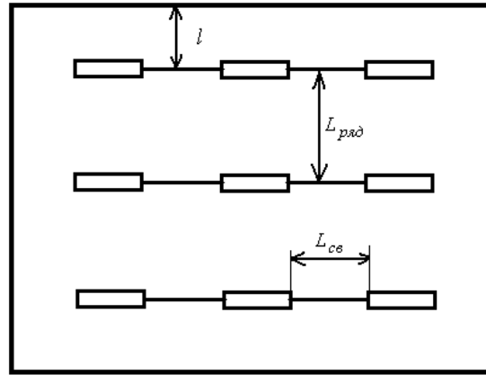
Рис.3. Расположение светильников с люминесцентными лампами.
