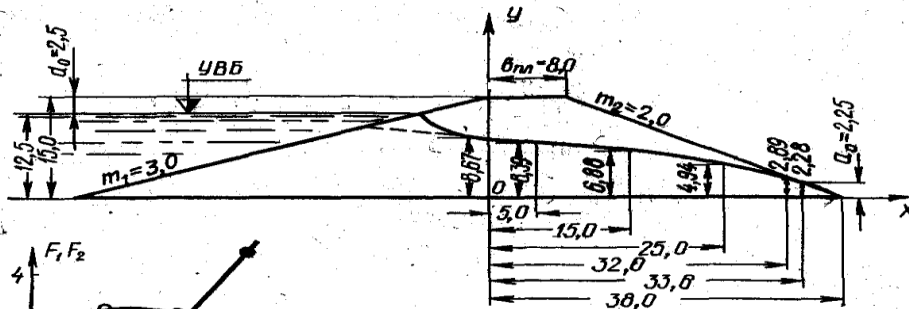
Расчетная схема фильтрации через однородную земляную плотину на водонепроницаемом основании, без дренажа и при отсутствии воды в нижнем бьефе.
