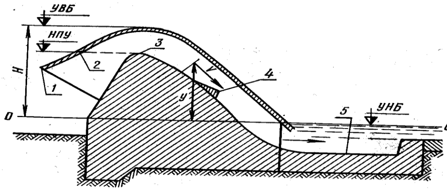
8.2 Расчетная схема сифонного водосброса. 1 – козырек; 2 – воздушное отверстие; 3 – гребень сифона; 4 – гусек; 5 – водобойный колодец.
