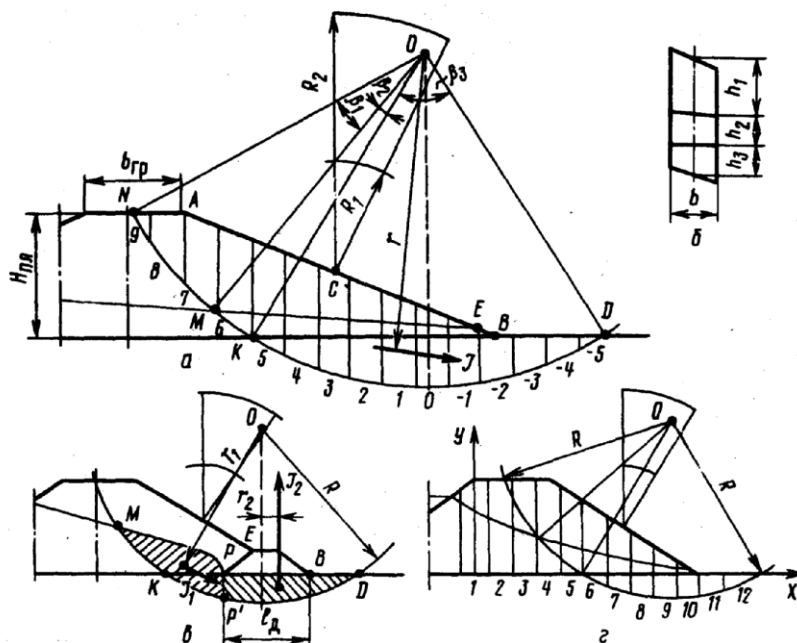
Рис.7.1 Расчетные схемы устойчивости низового откоса: а — при отсутствии дренажа; б — составные части отсека; в — при наличии дренажа; г — для расчета с применением ЭВМ.
