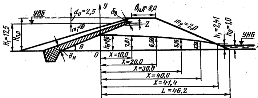
6.4 Расчетная схема фильтрации через земляную плотину с экраном на водопроницаемом основании без дренажа при наличии воды в нижнем бьефе.
