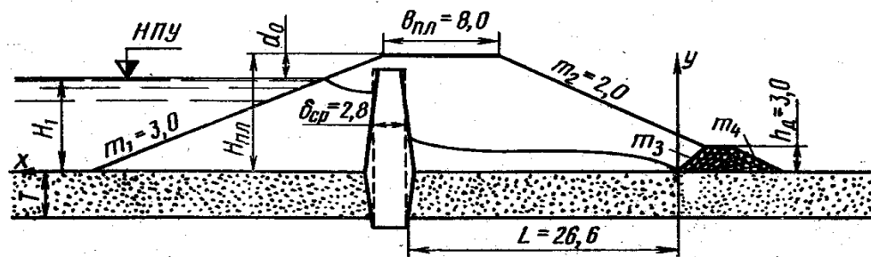
Расчетная схема фильтрации через земляную плотину с ядром и дренажем на водопроницаемом основании при отсутствии воды в нижнем бьефе.
