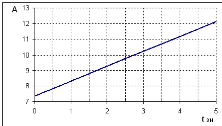
Рис. 19. График зависимости амплитуды А от зоны нечувствительности t_{зн} .
