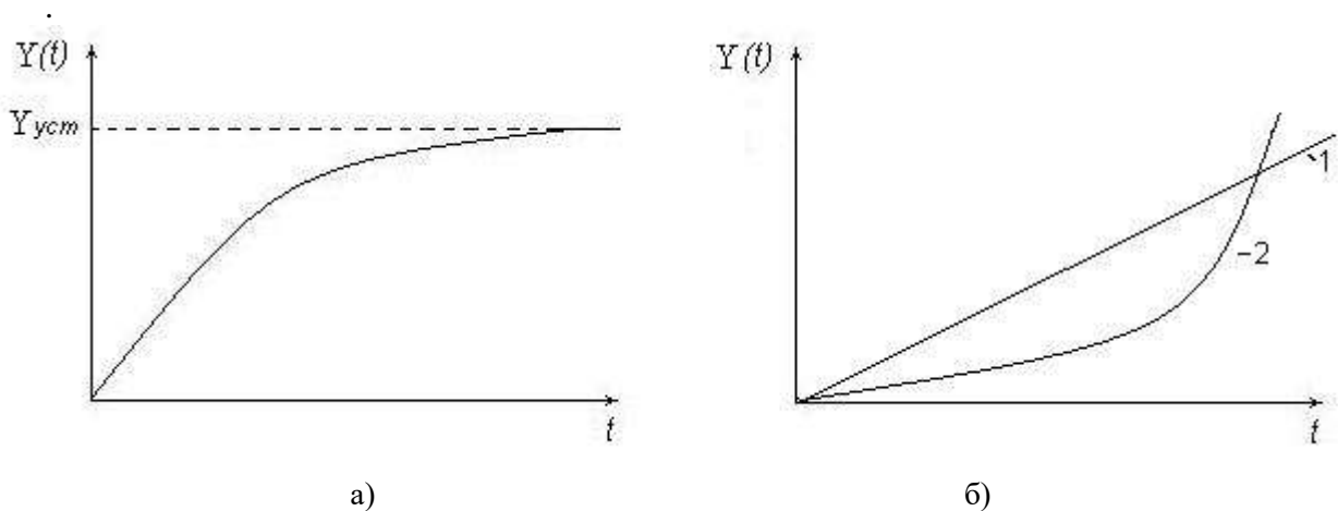
Рис. 4. Переходные функции объектов: а- переходная функция статического объекта; б- переходные функции астатических объектов, линейный объект (прямая 1) и нелинейный (кривая 2).
