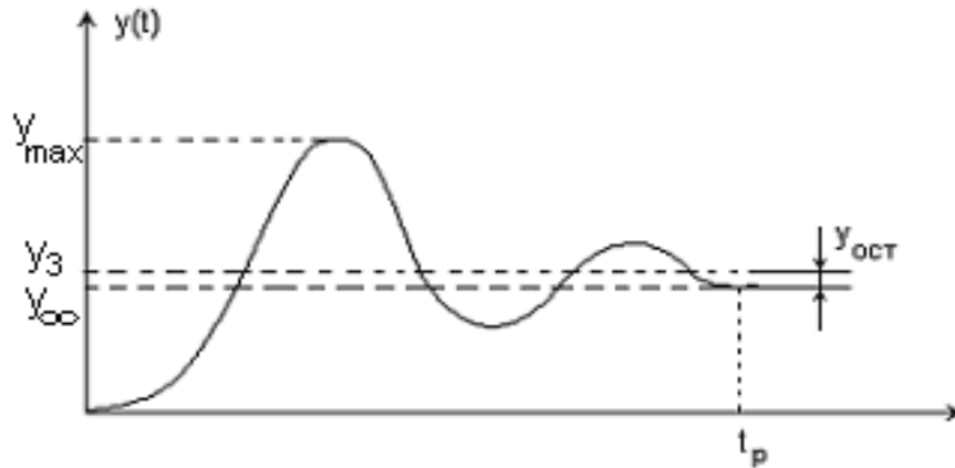
Рис.7. График переходного процесса регулирования АСР, здесь Y_з - заданное значение регулируемой величины; Y_{\infty} - установившееся значение регулируемой величины; Y_{\max} - максимальное значение регулируемой величины.
