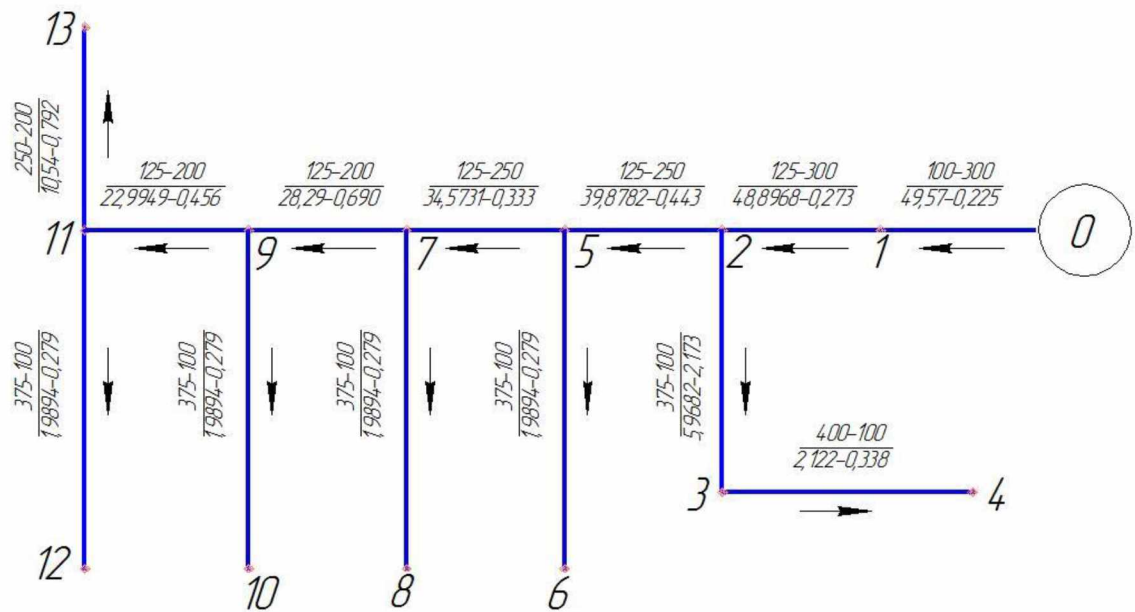
Рисунок 8 Гидравлическая схема сети \left(\frac{l-d}{Q-h}\right) , ( l – м; d – мм; Q – л/с; h – м)
