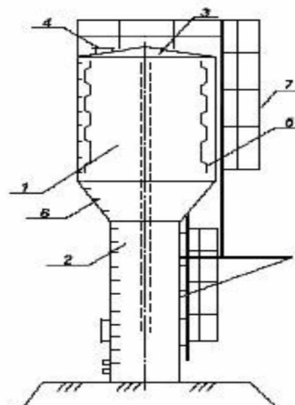
Рисунок 10 Водонапорная башня
