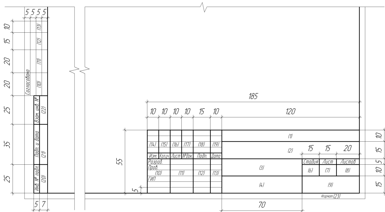
Форма 5а. Основная надпись листов рабочих чертежей.
