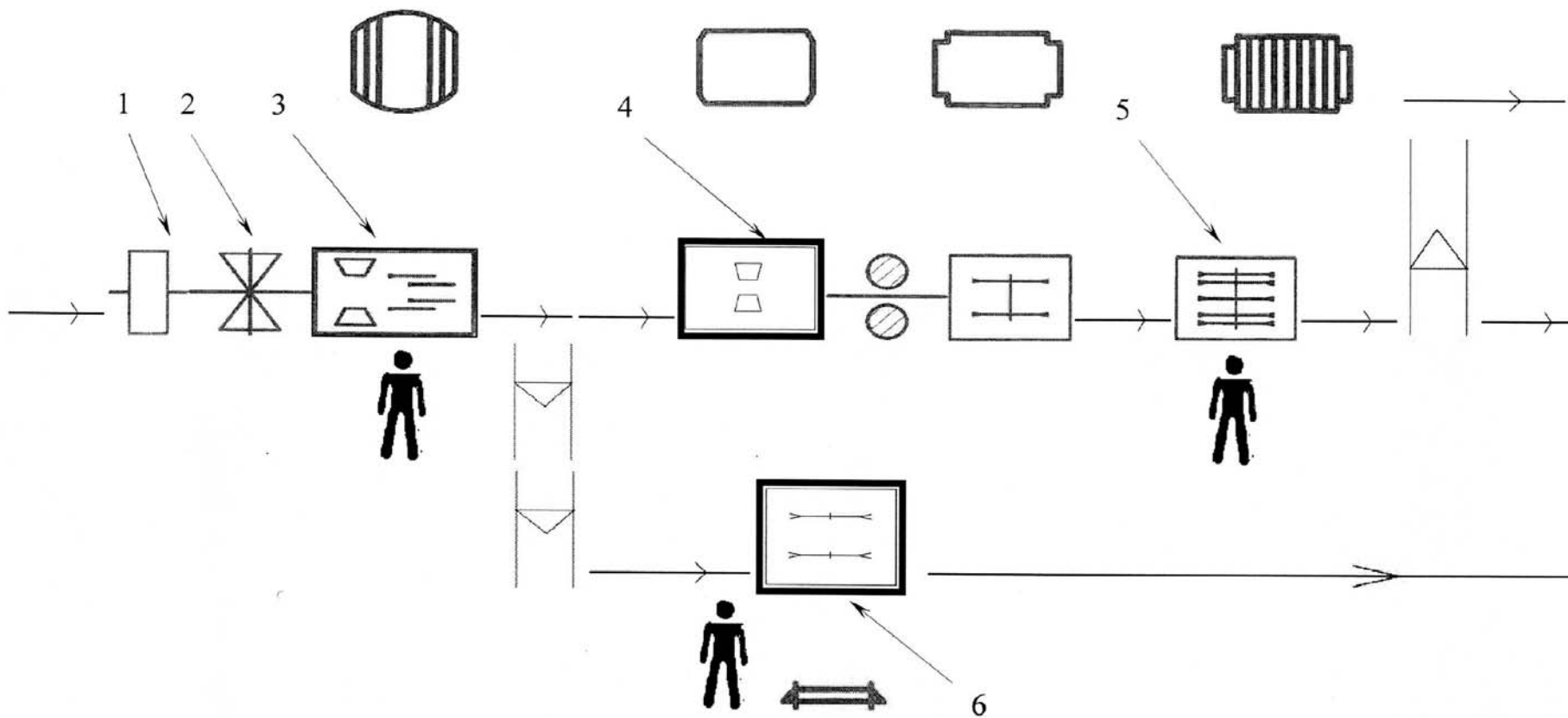
1 – трехмерный сканер; 2 – оптимизатор положения бревен; 3 – фрезерно-ленточнопильный агрегат (4-пильный); 4 – фрезерно-брусующий агрегат с профилирующим узлом обрезки кромок; 5 – многопильный круглопильный станок; 6 – обрезной станок.
