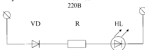
Рис.1. Схема подключения светодиода.
